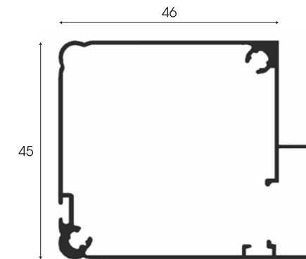
Cassonetto
