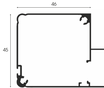
Cassonetto
